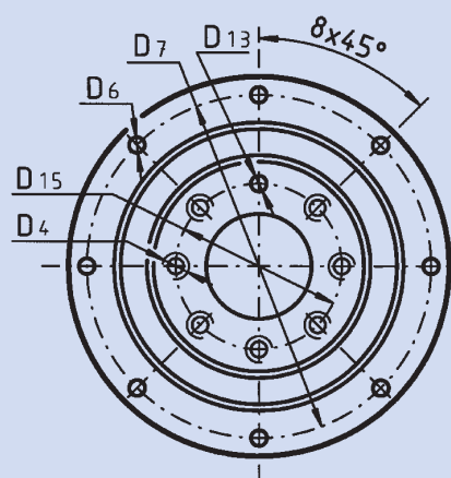
Typ MPG 02 Ansicht / View W:
