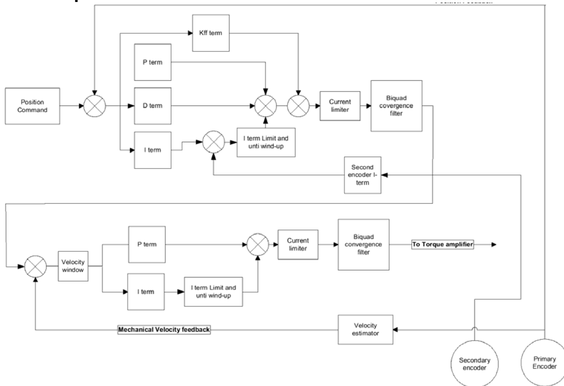
Диаграмма регулятора положения и скорости 940
